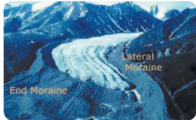
Fig. 3.34 : Glacial moraines
