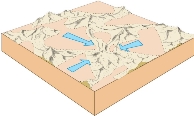
Fig. 3.27 : Star dunes
