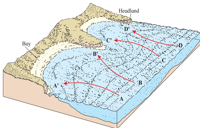
Fig. 3.8 : Wave refraction
