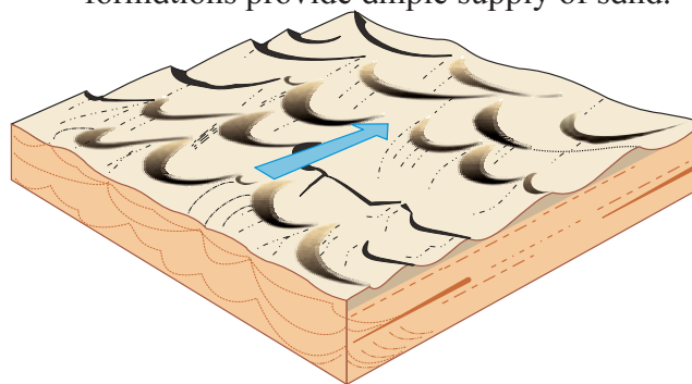
Fig. 3.24 : Transverse dunes
