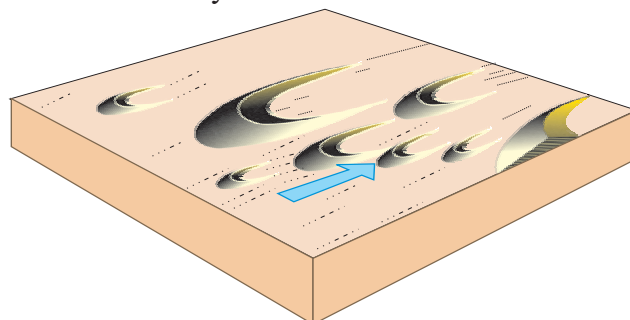
Fig. 3.25 : Barchan dunes
