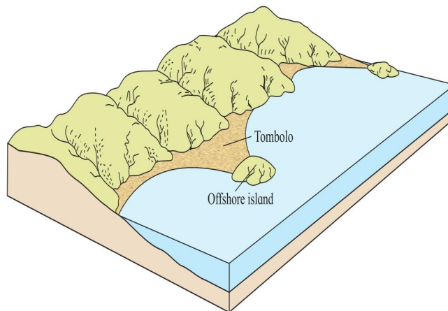
Fig. 3.14 : Tombolo
